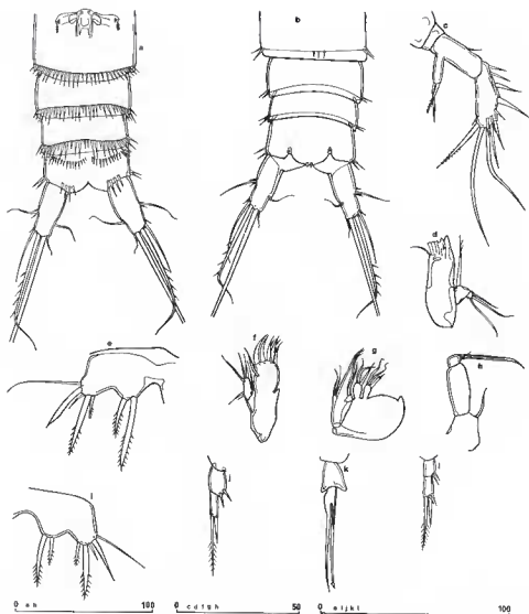
FIG. 3. — Ceuthonectes vievilleae n. sp. a : abdomen ♀, vue ventrale ; b : abdomen ♀, vue dorsale ; c : A_3 ♀ ; d : mandibule ♀ ; e : P_2 ♀ ; f : maxillule ♀ ; g : maxille ♀ ; h : maxillipède ♀ ; i : P_3 ♂ ; j : endopodite P_2 ♂ ; k : endopodite P_3 ♂ ; l : endopodite P_4 ♂. (Échelle micrométrique.)
